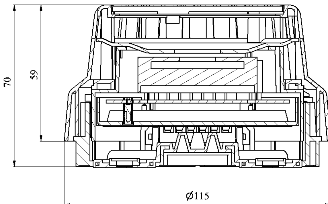
Rys. 1 Konstrukcja mechaniczna sygnalizatora SAW-6000.
